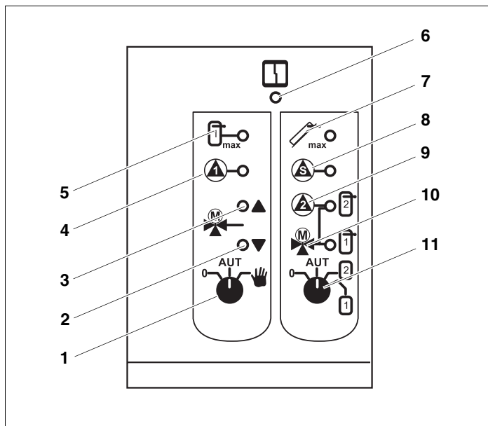
Рис. 1 Фронтальная панель функционального модуля FM 443
