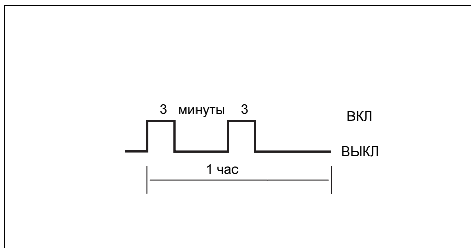
Рис. 10 Схема работы циркуляционного насоса при заводской настройке 2
