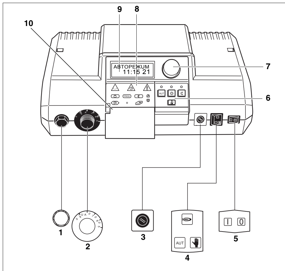
Рис. 1 Элементы управления Logamatic 2107 и Logamatic 2107 М
