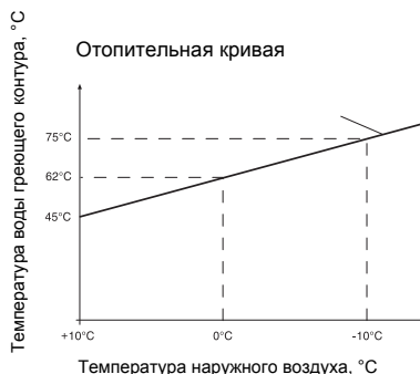
Рис. 11 Тест отопительной кривой
