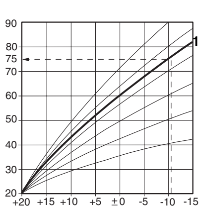
Рис. 8 Определение отопительной кривой
