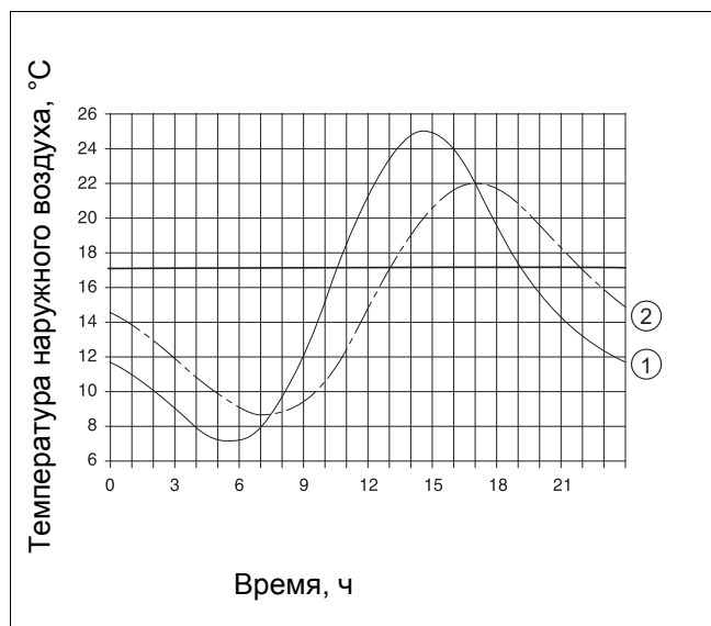
Рис. 7 Термическое запаздывание
