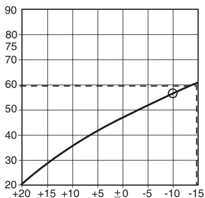
Рис. 9 Определение отопительной кривой
